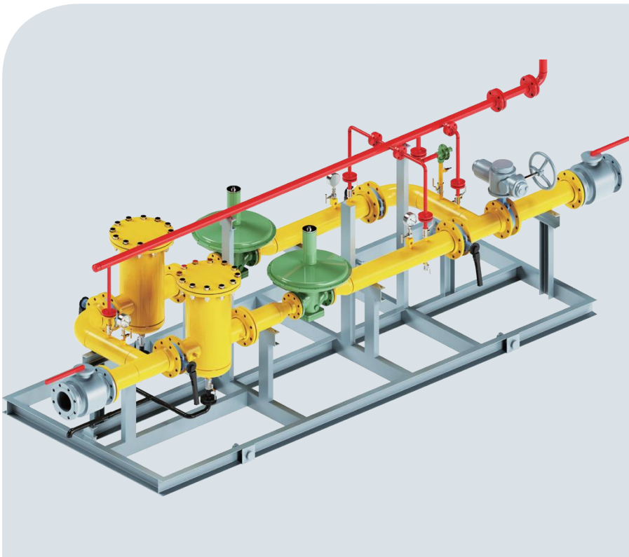
中低压调压柜
